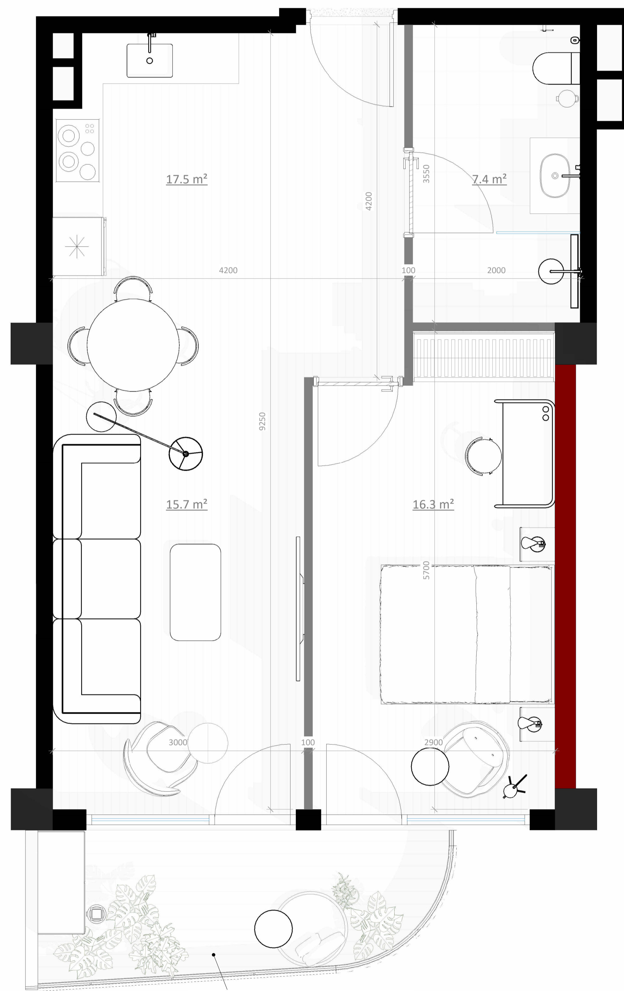
სართ. სიმაღლე | FLOOR H 35.1 m
